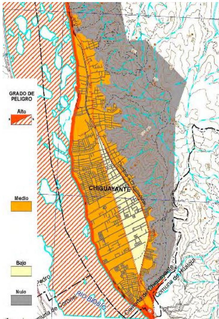
Imagen 9: Carta geo ambiental: “Peligro de licuefacción: área Concepción-Talcahuano-Hualpén-Chiguayante”. SERNAGEOMIN
